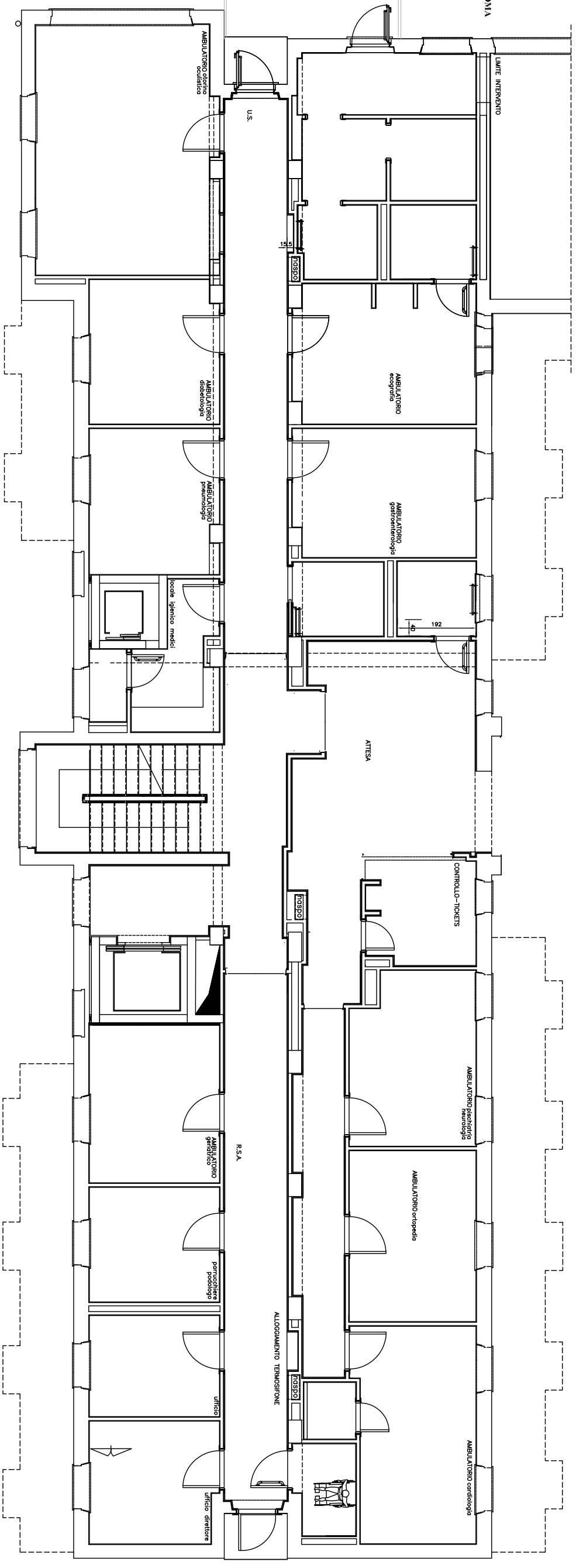
PIANTA PIANO PRIMO
